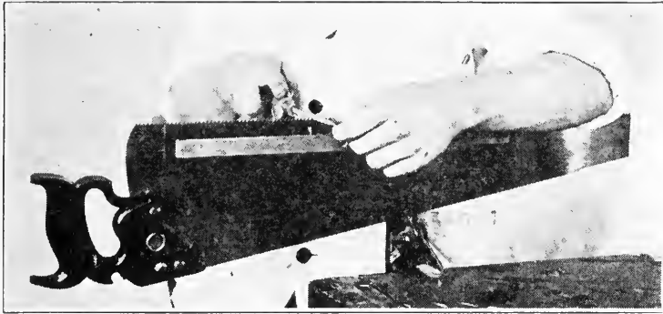
FIG. 112. FILING A RIP-SAW.
